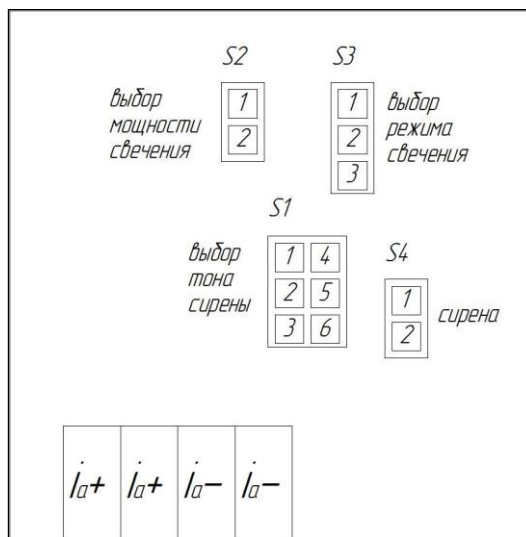
Рисунок 1 – Схема расположения контактов подключения цепи питания и штыревых контактов выбора режимов работы
