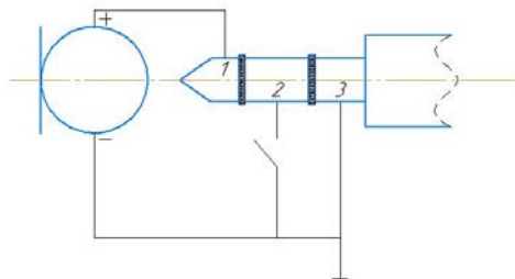
Рис.2. Схема подключения
