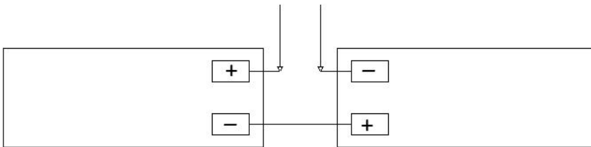
Рисунок 1. Схема подключения АКБ
