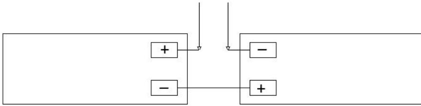
Рис. 2 Схема подключения АКБ
